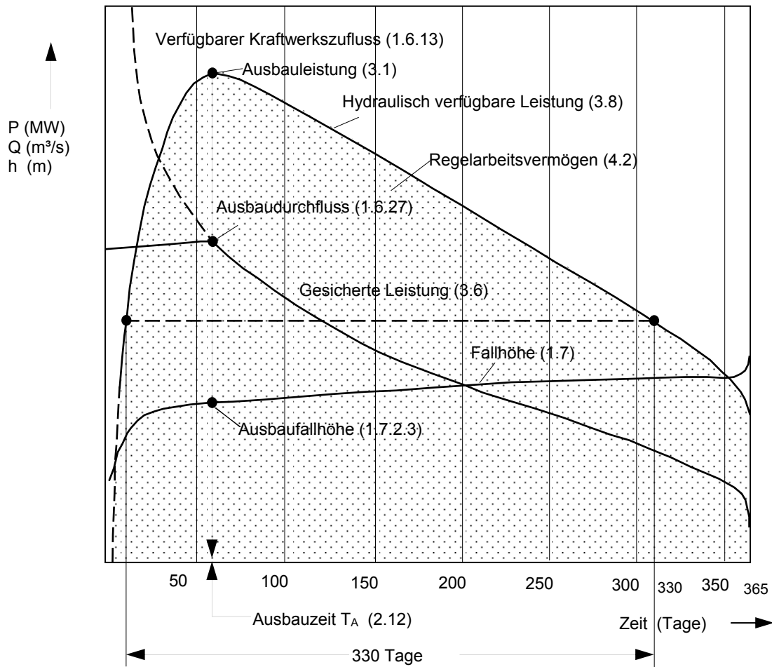
Bild 11: Werkleistungsplan eines Laufwasserkraftwerks
